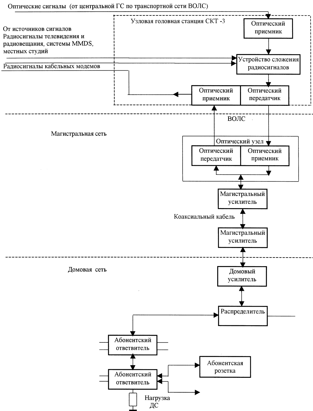
Рисунок 4.3 — Структурная схема городской кабельной распределительной сети СКТ-3
