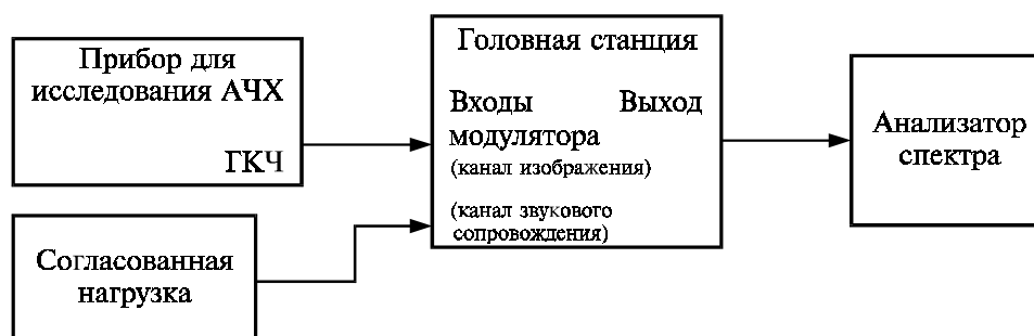
Рисунок 7.20 — Структурная схема для определения характеристики боковых полос
