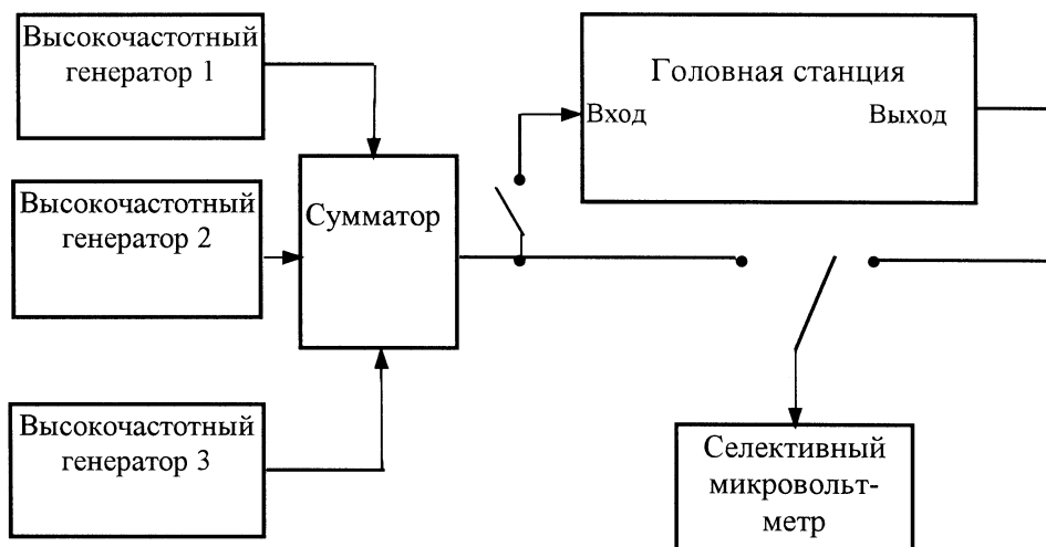
Рисунок 7.12 — Структурная схема для определения отношения радиосигнала изображения к одночастотной помехе комбинационных частот третьего порядка ИМА_{III(K)}
