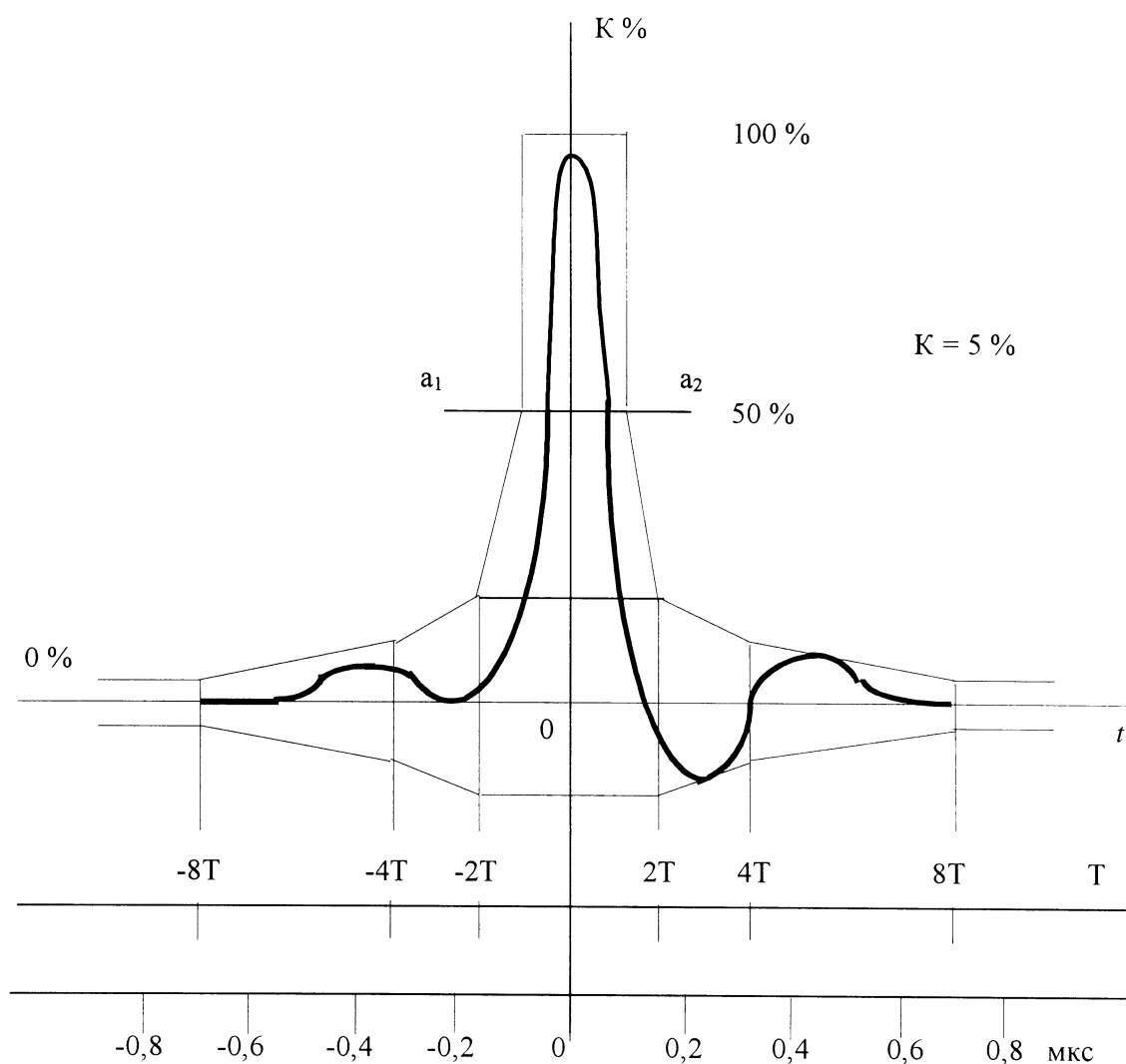
Рисунок 7.3 — Осциллограмма 2Т-импульса измерительного сигнала № 2 (ГОСТ 18471)
