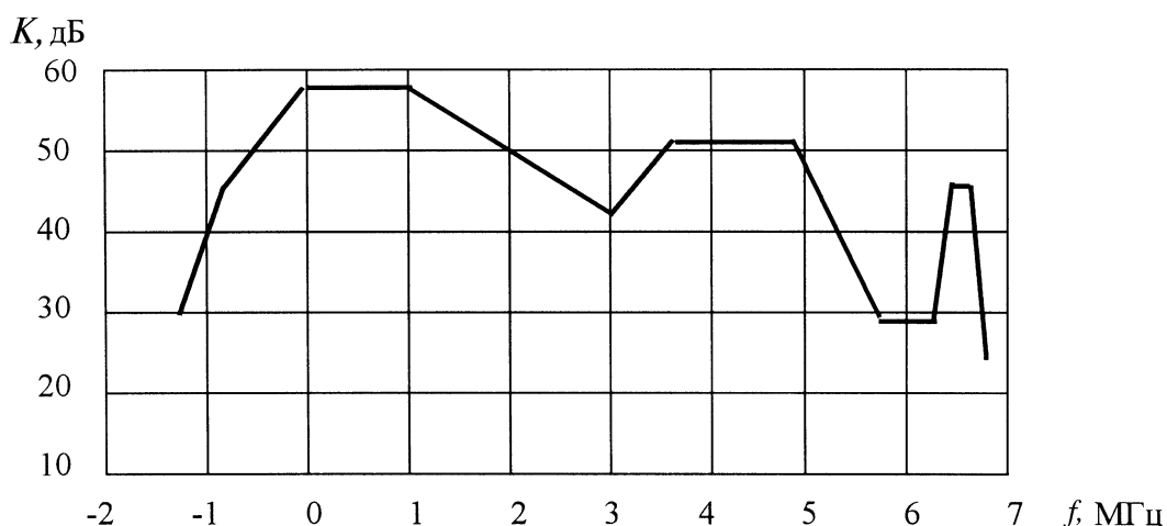
Рисунок 5.1 — Кривая защитных отношений для системы вещательного телевидения
