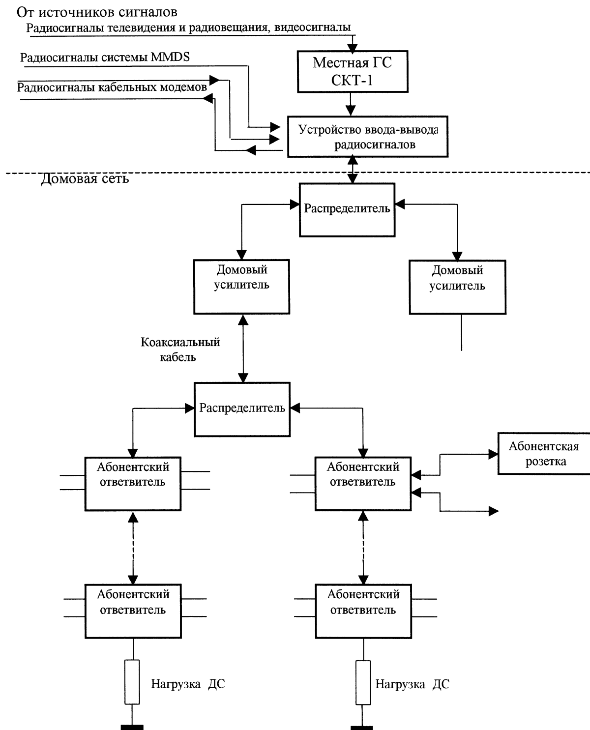
Рисунок 4.1 — Структурная схема местной кабельной распределительной сети СКТ-1
